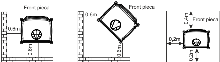
Rysunek 3. Bezpieczne odległości ustawienia pieca od ścian, mebli w pomieszczeniach.
